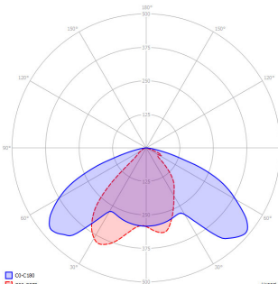
Lichtverteilung L5
