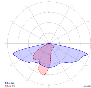
Lichtverteilung L9
