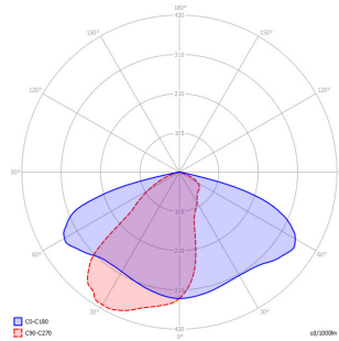
Lichtverteilung L5
