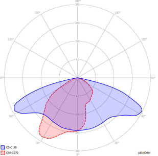
Lichtverteilung L7
