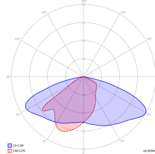
Lichtverteilung L8
