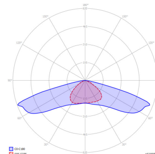
Lichtverteilung L6
