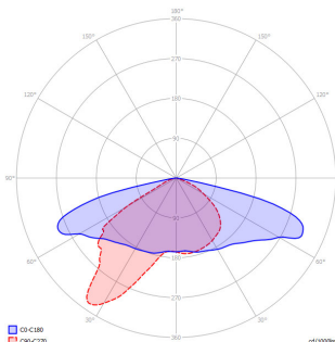
Lichtverteilung L4
