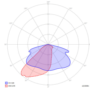
Lichtverteilung L6
