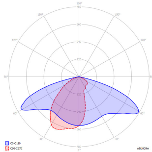
Lichtverteilung L4
